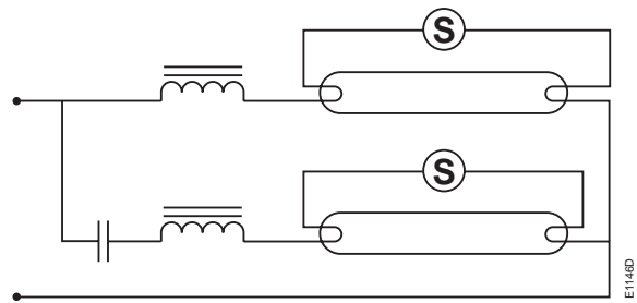
Последовательная компенсация при спаренной установке
