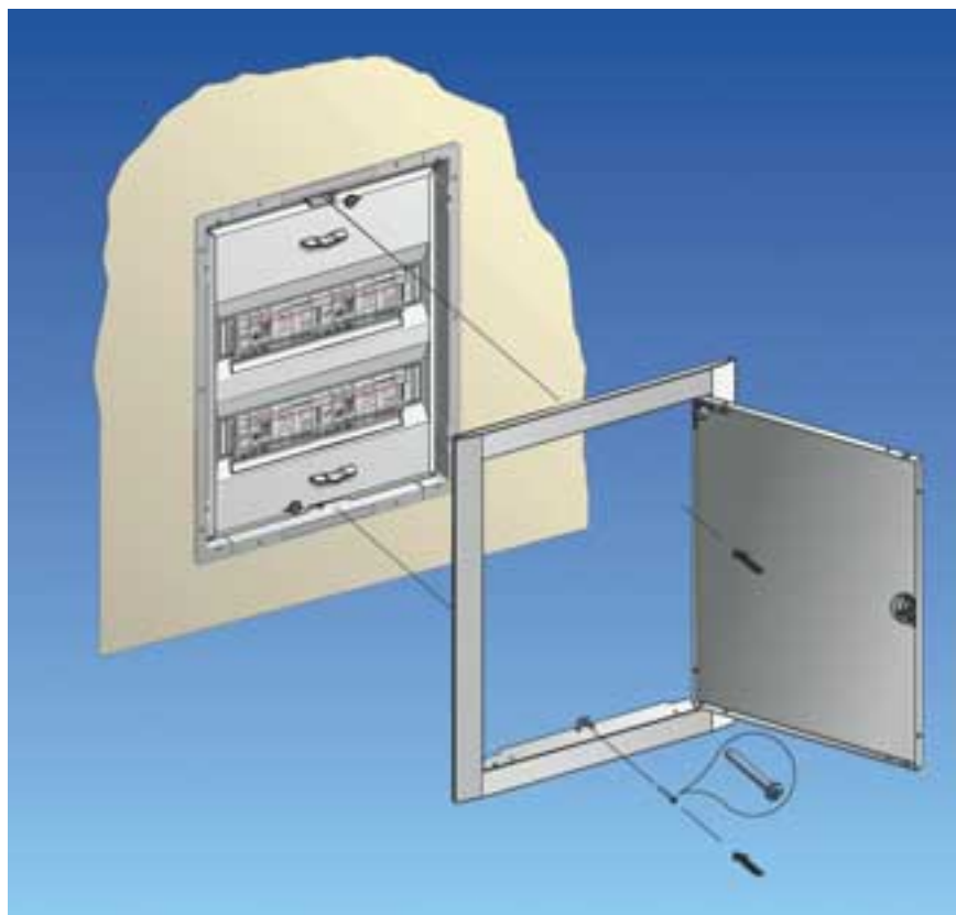
Легко монтируемая рама с дверцей. Возможность установки заподлицо с оштукатуренной поверхностью стены. Пломбируемая защитная крышка фиксируется поворотными (на 90°) замками.
